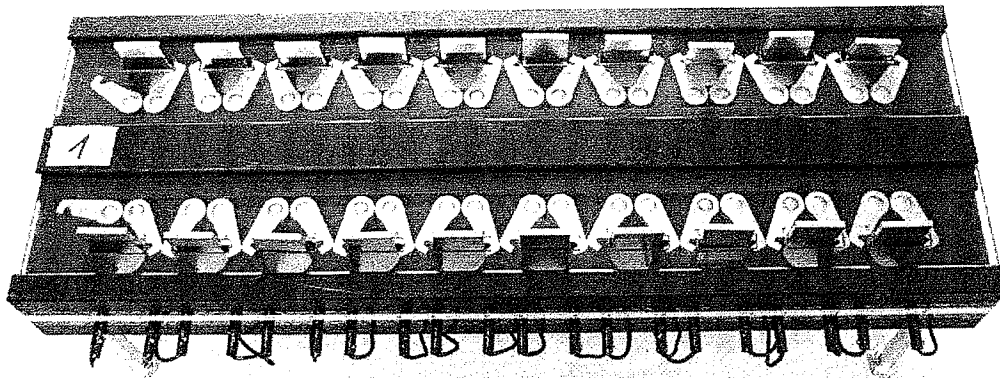
Bild 1: WSR-Verspannvorrichtung
