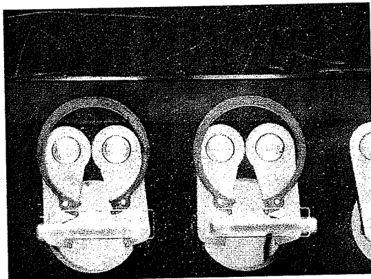
Bild 8: Verspannte WSR
