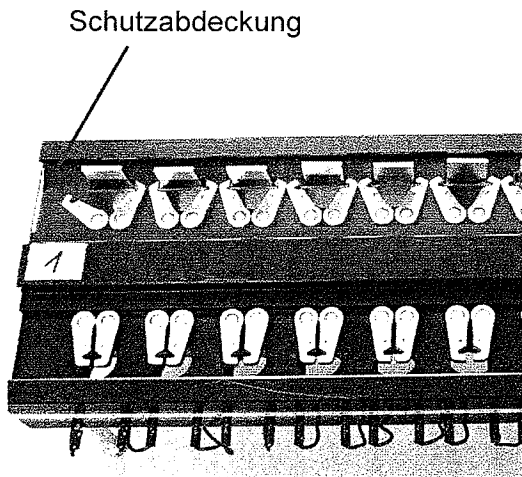
Bild 2: Abgenommene Schutzabdeckung
