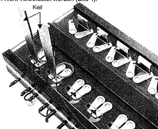
Bild 4: Positionierte Keile
