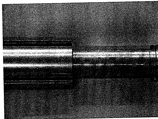
Bild 7: Mitte der Kontrollbohrung in Deckung mit der Kante der Führungshülse
